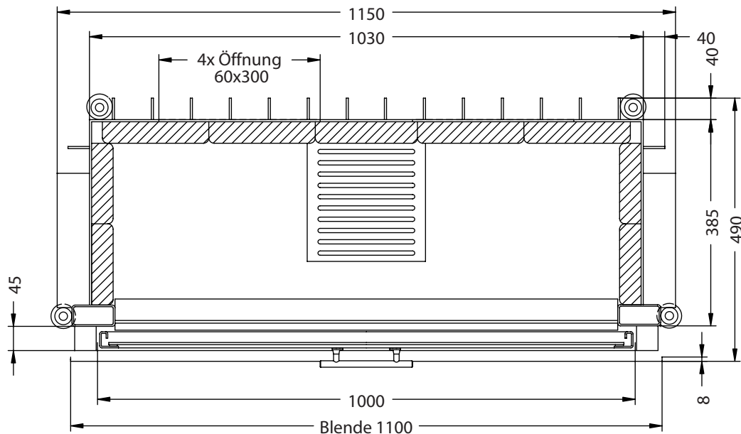
Horizontalschnitt M~1:10
