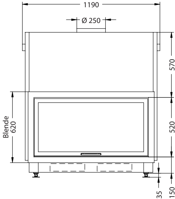
Vorderansicht M~1:20
