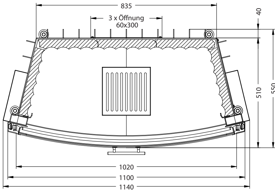
Horizontalschnitt M~1:10
