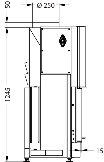
Seitenansicht M~1:20
