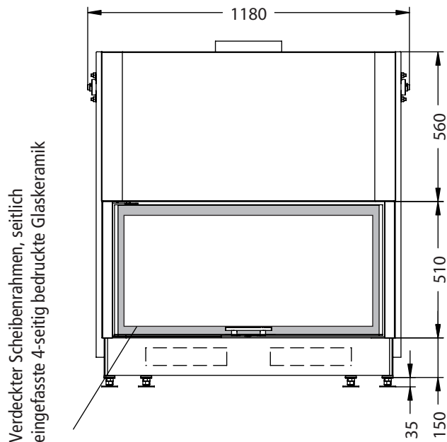
Vorderansicht M~1:20
