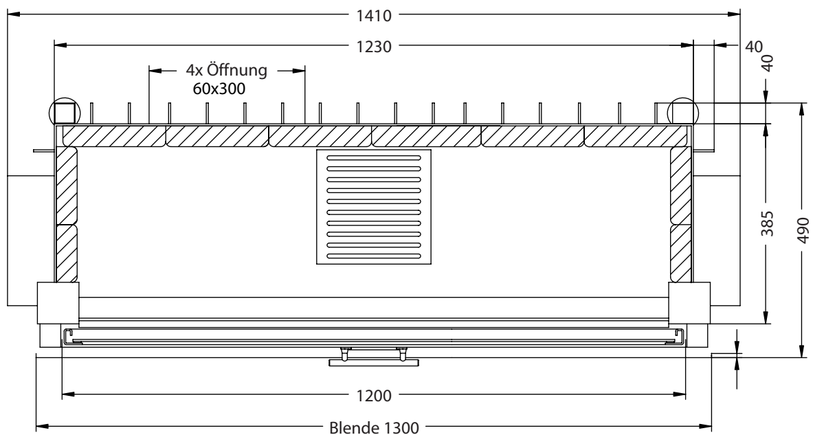
Horizontalschnitt M~1:10
